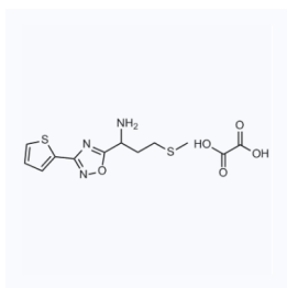
1144656 CAS: 1820649-57-7
