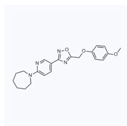
1145511 CAS: 1358349-74-2
