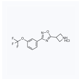
1145610 CAS: 1351584-79-6
