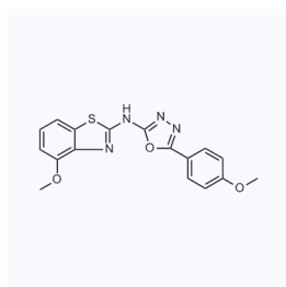
1103780 CAS: 862974-25-2
