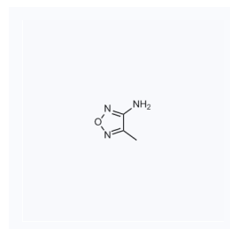
1115595 CAS: 17647-70-0
