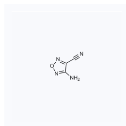
1151094 CAS: 156463-85-3
