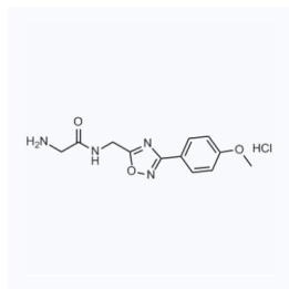
1145281 CAS: 1441889-72-0
