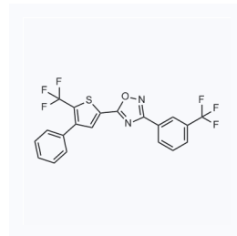
1027509 现货 CAS: 256414-75-2
