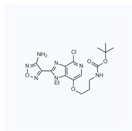
1057372 CAS: 1052112-24-9
