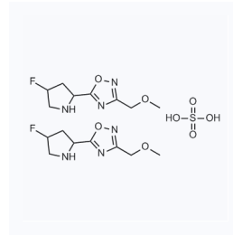
1143983 CAS: 2097936-55-3
