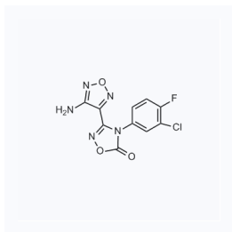
1085849 CAS: 1204669-80-6
