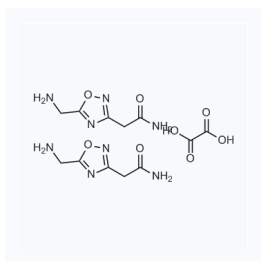
1144662 CAS: 1820639-54-0
