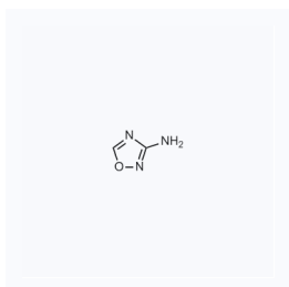
1155717 CAS: 39512-64-6
