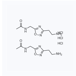
1144633 CAS: 1820673-59-3
