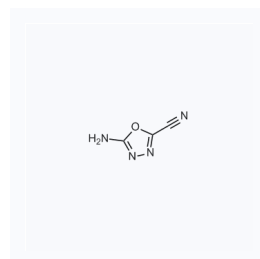
1149645 CAS: 134318-57-3
