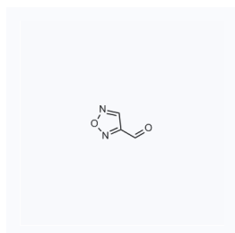
1151035 CAS: 1485710-88-0
