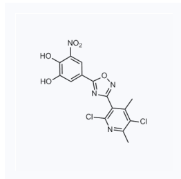
1080978 现货 CAS: 952091-17-7
