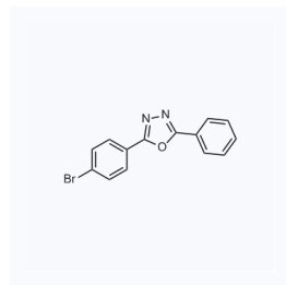
1133825 CAS: 21510-43-0
