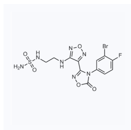
1060691 现货 CAS: 1204669-70-4
