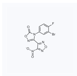
1113016 CAS: 2019140-71-5
