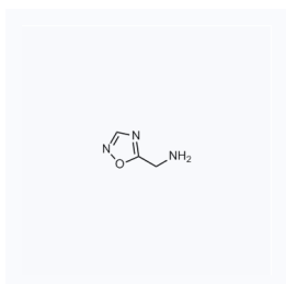
1154368 CAS: 258526-20-4
