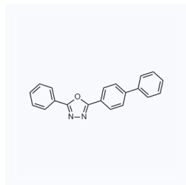
1044880 CAS: 852-38-0
