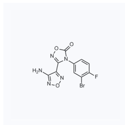
1060687 现货 CAS: 914471-43-5
