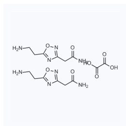
1144676 CAS: 1820614-77-4
