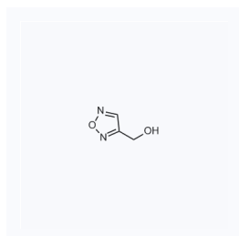
1151032 CAS: 79552-35-5
