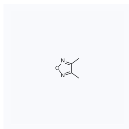
1151092 CAS: 4975-21-7
