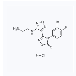
1060689 现货 CAS: 1204669-67-9
