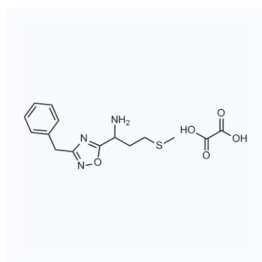
1144614 CAS: 1820703-53-4
