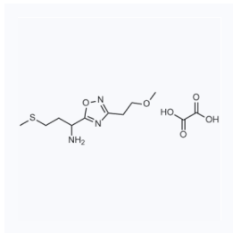
1144605 CAS: 1820705-96-1
