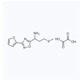
1144654 CAS: 1820650-54-1
