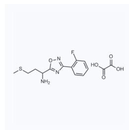
1144604 CAS: 1820705-98-3
