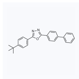
1022144 CAS: 15082-28-7
