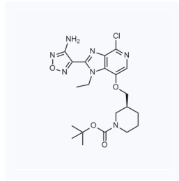
1057378 CAS: 937174-74-8
