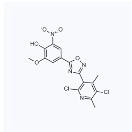
1080503 现货 CAS: 1391712-50-7
