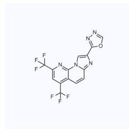
1126462 现货 CAS: 691868-88-9
