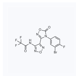
1060688 CAS: 914471-60-6
