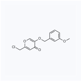
1146020 CAS: 1248907-44-9
