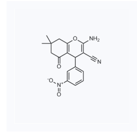
1181406 CAS: 144036-36-2
