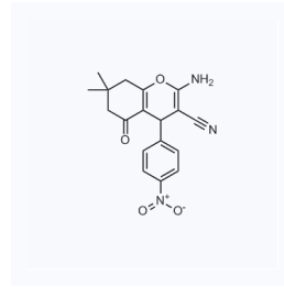
1181408 CAS: 144036-35-1
