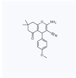
1181405 CAS: 129354-36-5
