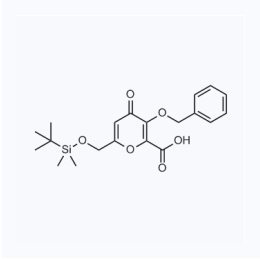
1122152 CAS: 895134-29-9
