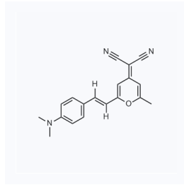
1034225 CAS: 51325-91-8
