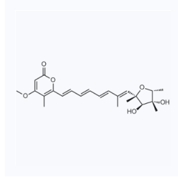
1027439 CAS: 25425-12-1
