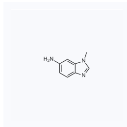
1067888 CAS: 26530-93-8
