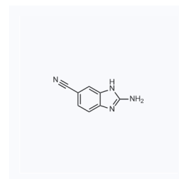
1115683 CAS: 63655-40-3
