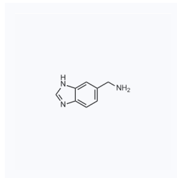
1182307 CAS: 164648-60-6
