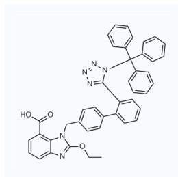
1064465 CAS: 139481-72-4
