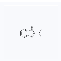
1187655 CAS: 5851-43-4
