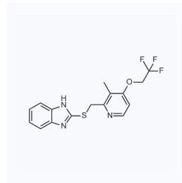
1015410 CAS: 103577-40-8
