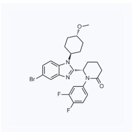
1172095 现货 CAS: 2222964-03-4
