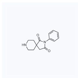
1057865 现货 CAS: 64097-70-7
