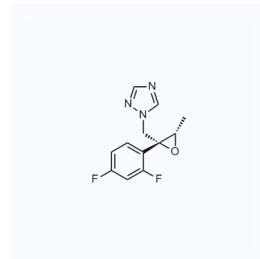
1066781 现货 CAS: 127000-90-2
