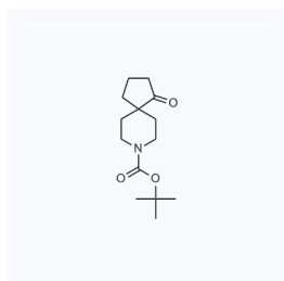
1050421 现货 CAS: 191805-29-5
