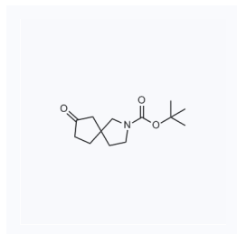
1118773 现货 CAS: 1319716-42-1
