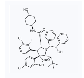
1060515 现货 CAS: 1303609-36-0
