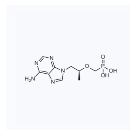
1182532 现货 CAS: 147127-19-3
