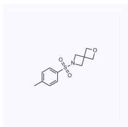
1057885 现货 CAS: 13573-28-9
