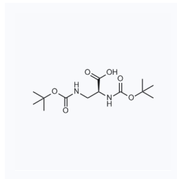
1170445 现货 CAS: 88971-40-8
