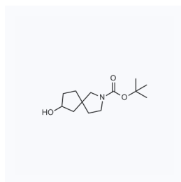
1118777 现货 CAS: 1319716-41-0
