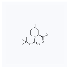
1058084 现货 CAS: 796096-64-5
