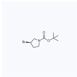
1036229 现货 CAS: 569660-97-5
