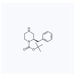
1052540 现货 CAS: 947684-78-8
