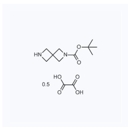
1053092 现货 CAS: 1041026-71-4
