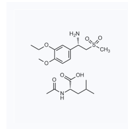
1060490 现货 CAS: 608141-43-1
