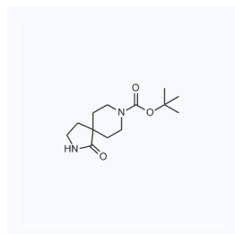
1051266 现货 CAS: 268550-48-7
