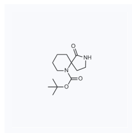
1067085 现货 CAS: 1221818-08-1
