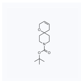
1057697 现货 CAS: 374795-40-1
