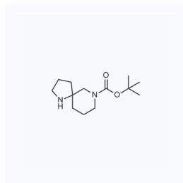
1070663 现货 CAS: 939793-21-2
