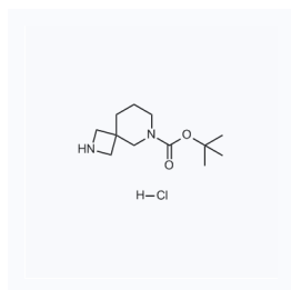
1105957 现货 CAS: 1279844-25-5
