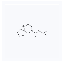
1106058 现货 CAS: 886766-37-6
