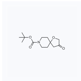
1069825 现货 CAS: 954236-44-3
