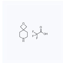
1048427 现货 CAS: 1257381-44-4
