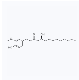
1026703 现货 CAS: 23513-15-7
