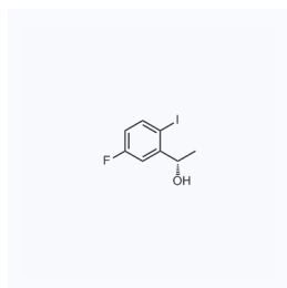
1149240 现货 CAS: 1454847-96-1
