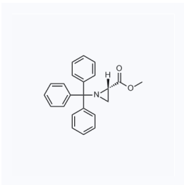
1041948 现货 CAS: 75154-68-6
