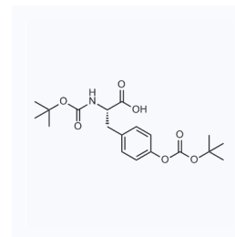
1171192 现货 CAS: 20866-48-2
