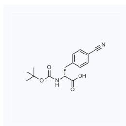
1021755 现货 CAS: 146727-62-0
