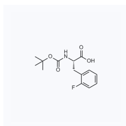
1017457 现货 CAS: 114873-00-6
