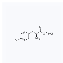
1064234 现货 CAS: 99359-32-7
