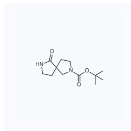
1051070 现货 CAS: 1194376-44-7
