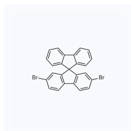
1023555 现货 CAS: 171408-84-7
