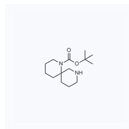
1070533 现货 CAS: 960294-18-2
