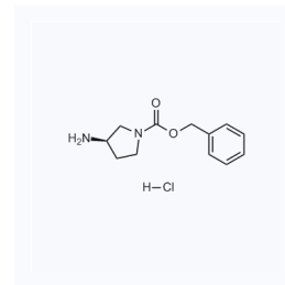
1045254 现货 CAS: 870621-17-3
