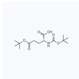
1015616 现货 CAS: 104719-63-3
