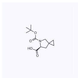
1060314 现货 CAS: 1129634-44-1
