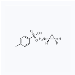
1063545 现货 CAS: 143062-84-4
