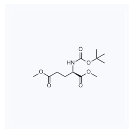
1066744 现货 CAS: 130622-05-8
