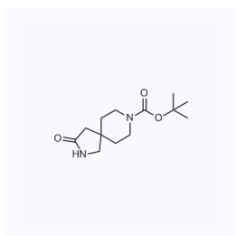
1057864 现货 CAS: 169206-67-1
