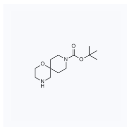
1063307 现货 CAS: 930785-40-3
