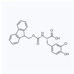
1064241 现货 CAS: 478183-58-3
