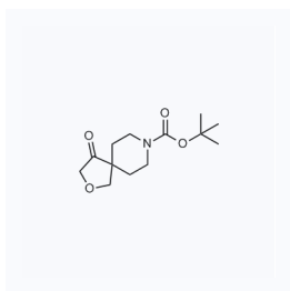
1159664 现货 CAS: 1801766-68-6
