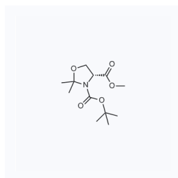
1050385 现货 CAS: 95715-86-9
