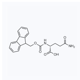
1017265 现货 CAS: 112898-00-7
