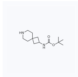
1112261 现货 CAS: 147611-03-8
