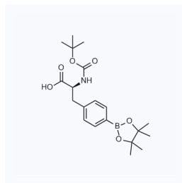
1061211 现货 CAS: 216439-76-8
