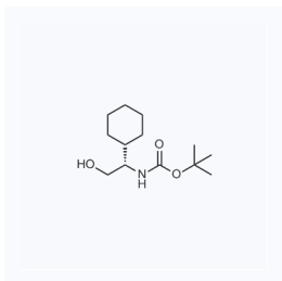
1016065 现货 CAS: 107202-39-1
